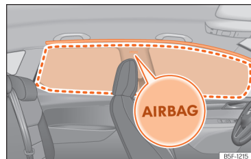
SL. 30 Mjesto ugradnje i područje širenja zračnog jastuka za glavu.
