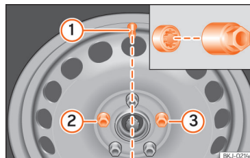
Sl. 227 Zamjena kotača: ventil gume ① i mjesto ugradnje vijka kotača sa zaštitom od krađe ② ili ③.
