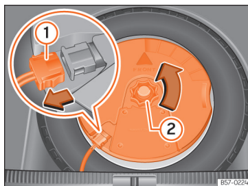
Sl. 222 U prtljažniku: demontiranje subwoofera.
