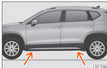
Sl. 228 Mjesta za postavljanje dizalice vozila.
