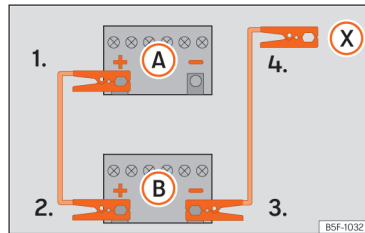
Sl. 193 Plan priključivanja za vozila bez start-stop sustava.
