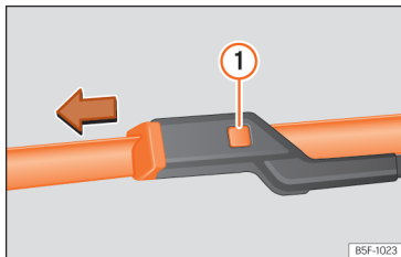
SL. 191 Zamjena prednjih metlica brisača.
