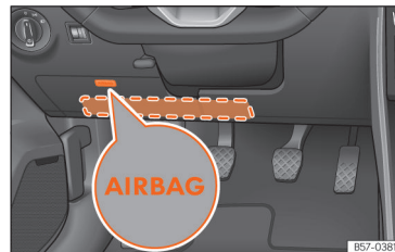
SL. 31 Na vozačevoj strani: mjesto ugradnje zračnog jastuka za koljena.
