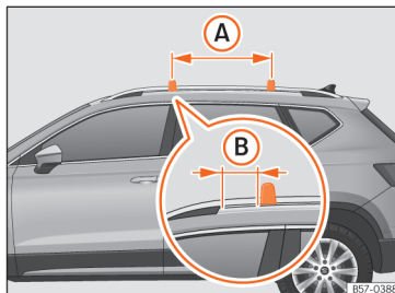
SL. 180 Pričvrstne točke poprečnih šipki za krovni nosač prtljage.
