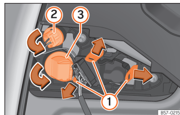
Sl. 206 Demontaža držača žaruljice.
