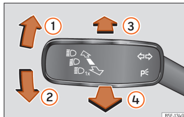
Sl. 81 Ručica za žmigavce i duga svjetla.
