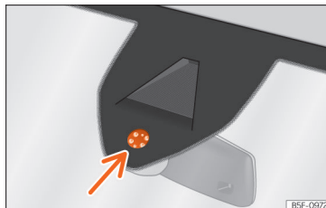
Sl. 91 Senzor za vlagu i temperaturni senzor na vjetrobranskom staklu.
