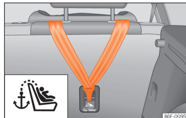
SL 38 Stražnja strana stražnje klupe: pričvrstne ušice za Top Tether pričvrstni pojas.
