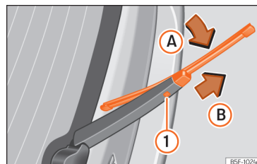
SL. 192 Zamjena metlice brisača stražnjeg stakla.
