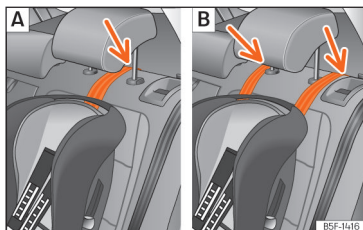
Sl. 39 Stražnja sjedala: namještanje i ugradnja uz korištenje Top Tether pojasa.
