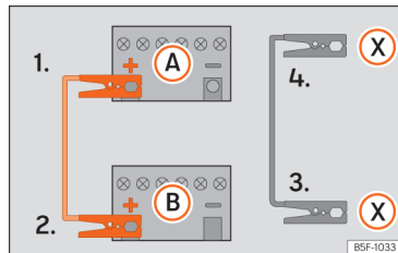
Sl. 194 Plan priključivanja za vozila sa start-stop sustavom.
