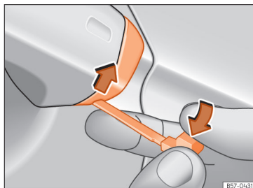
Sl. 53 Ručica vozačkih vrata: odizanje poklopca.
