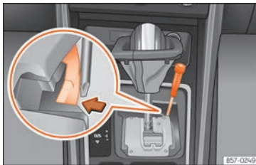
Sl. 88 Ručica automatskog mjenjača: deblokiranje u nuždi iz položaja za parkiranje
