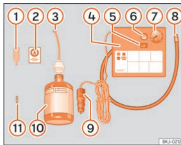
SL. 201 Prikaz principa: sastavni dijelovi kompleta za popravak guma
