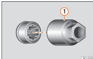
SL. 195 Vijak kotača sa zaštitom od krađe s kavicom i adapter
