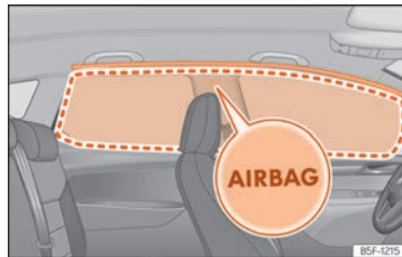
SL 31 Mjesto ugradnje i područje širenja zračnog jastuka za glavu.
