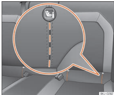
SL 35 Stražnje sjedalo: urezani prorezi za pristup ISOFIX/i-Size pričvršnim ušicama.
