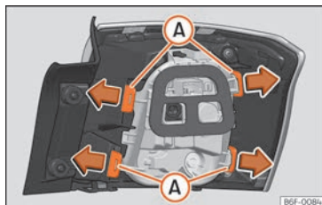
Sl. 172 Pričvrstne omče na poledini stražnjeg svjetla.
