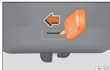
Sl. 56 Isječak iz prtljažnika: otključavanje u nuždi.
