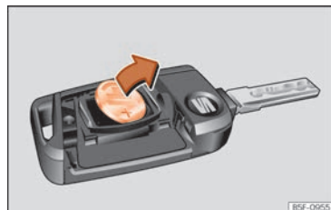
Sl. 46 Ključ vozila: vađenje baterije.
