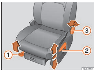
SL 61 Prednja sjedaća: manualno pomicanje sjedaća.
