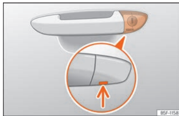
Sl. 51 Ručica vozačevih vrata: skriveni cilindar brave.
