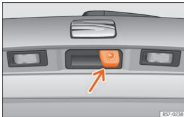
Sl. 113 U hvatištu stražnjeg poklopca: kamera za nadzor okoline.
