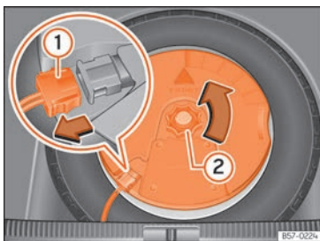
Sl. 218 U prtljažniku: demontiranje subwoofera.
