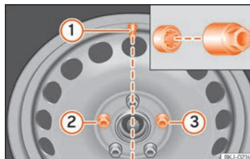
Sl. 223 Zamjena kotača: ventil gume ① i mjesto ugradnje vijka kotača sa zaštitom od krađe ② ili ③.
