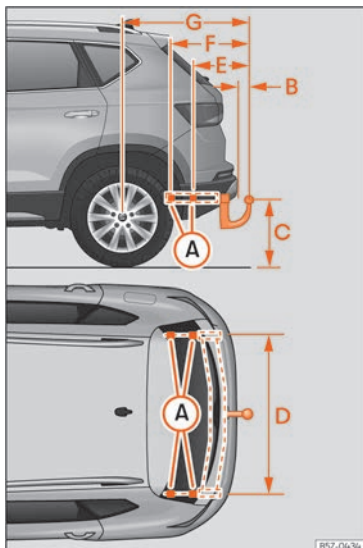
Sl. 183 Dimenzije i pričvrсна mjesta za naknadnu ugradnju mehanizma za vuču
