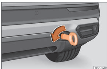
SL. 196 Na desnoj strani stražnjeg branika: Zavrnutu ušicu za vuču.
