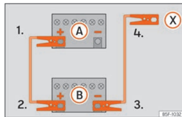
Sl. 191 Shema priključivanja za vozila bez start-stop sustava.
