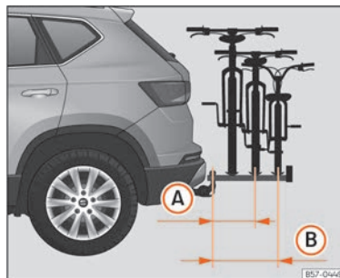
SL. 182 Shematski prikaz maksimalnog prevjesa tereta na nosaču za bicikl za dva ili tri bicikla.
