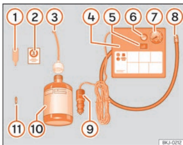
Sl. 227 Prikaz principa: sastavni dijelovi kompleta za popravak guma
