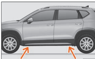
Sl. 224 Mjesta za postavljanje dizalice vozila.
