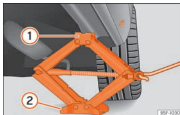
Sl. 225 Uzdužni nosač: postavljanje dizalice vozila.
