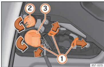
Sl. 202 Demontaža držača žaruljice.
