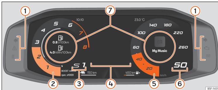
Sl. 2 Hibridna vozila: SEAT Digital Cockpit u instrumentnoj ploči (klasični prikaz).
