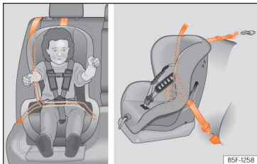
Sl. 47 Na stražnjim sjedalima: ugradnja dječjih sjedalice.
