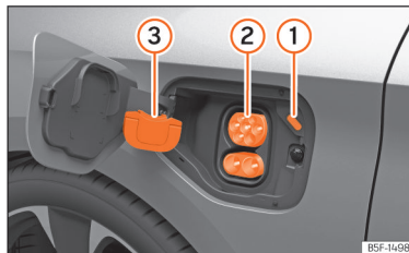
Sl. 60 Iza poklopca priključka za punjenje baterije straga desno: Priključak za punjenje.
