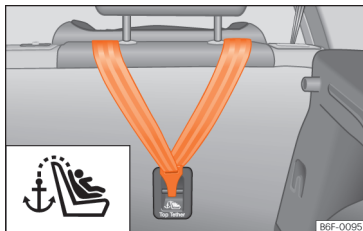
SL. 43 Stražnja strana stražnje klupe: pričvrсни ušice za Top Tether pričvrсни pojas.
