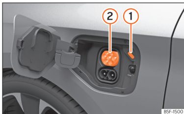
Sl. 58 Iza poklopca priključka za punjenje baterije srijeda lijevo: priključak za punjenje
