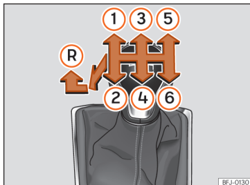
Sl. 123 Shema mijenjanja stupnjeva prijenosa kod 6-stupnjaskog ručnog mjenjača.
