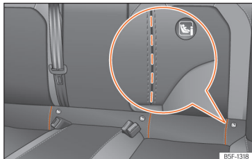
SL 40 Stražnje sjedalo: urezani prerezi za pristup ISOFIX/i-Size pričvršnim ušicama.
