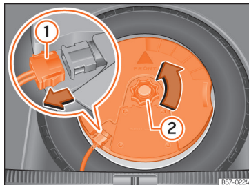
Sl. 242 U prtljažniku: demontiranje subwoofera.
