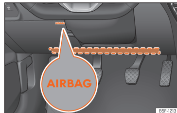
Sl. 35 Na vozačevoj strani: mjesto ugradnje zračnog jastuka za koljena.
