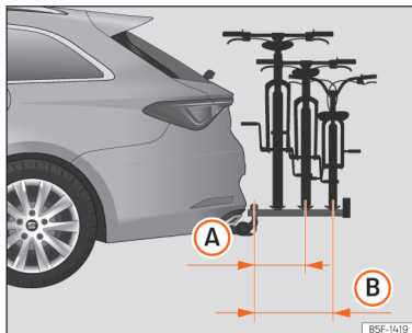
Sl. 203 Shematski prikaz maksimalnog prevjesa tereta na nosaču za bicikl za dva ili tri bicikla.
