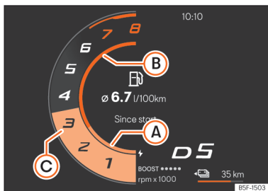
Sl. 5 Digitalni kombinirani instrument: Pokazivač stanja električnog pogona
