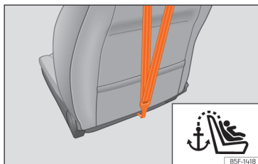
SL. 44 Stražnja strana naslona suvozačevog sjedala: mjesto pričvršćivanja za Top Tether pričvrсни pojas.
