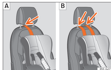
SL. 46 Suvozačvo sjedalo: namještanje i ugradnja uz korištenje Top Tether pojasa.
