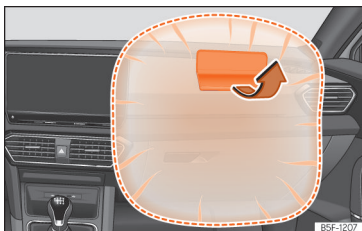
SL. 27 Suvozačev zračni jastuk u instrumentnoj ploči
