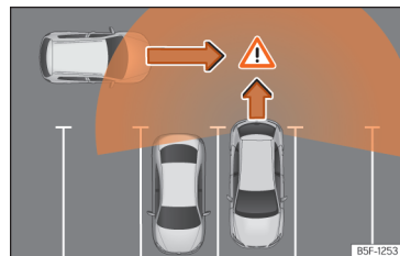
Sl. 124 Shematski prikaz potpore izlaska iz parkirnog mjesta: nadzirano područje vozila koje izlazi iz parkirnog mjesta.
