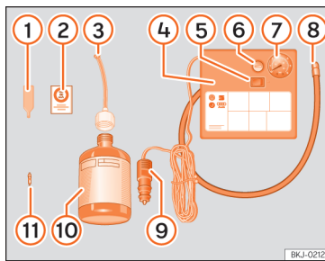
SL. 194 Prikaz principa: sastavni dijelovi kompleta za popravak guma
