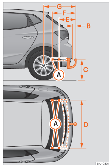
Sl. 146 Dimenzije i pričvrсна mjesta za naknadnu ugradnju mehanizma za vuču
