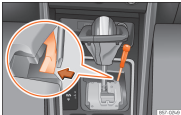
Sl. 90 Ručica automatskog mjenjača: deblokiranje u nuždi iz položaja za parkiranje
