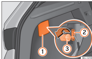
Sl. 163 Prtljažnik: pristup pričvršnom vijku stražnjeg svjetla
