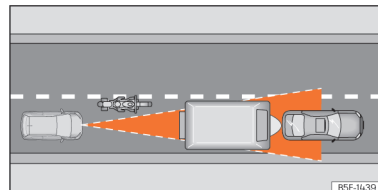
SL. 107 Vozač motocikla koji vozi ispred vašeg vozila izvan područja prepoznavanja radarskog senzora.
