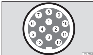
Sl. 143 Shematski prikaz: raspored zatika utičnih spojeva za struju prikolice.
