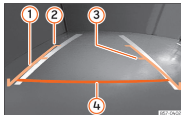
Sl. 123 Ekran infotainment sustava: Orijentacijske linije.
