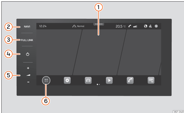
SL. 130 Pregled: jedinica za rukovanje.
