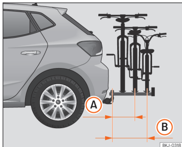
Sl. 145 Shematski prikaz maksimalnog prevjesa tereta na nosaču za bicikl za dva ili tri bicikla.
