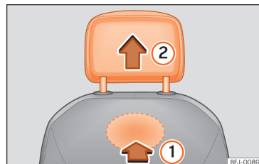
SL. 67 Demontaža naslona za glavu srijeda.
